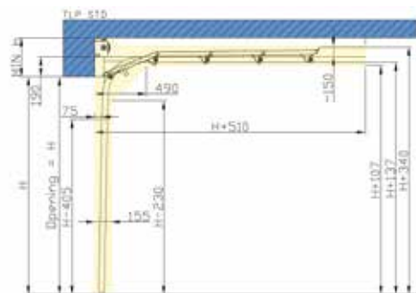
LHR-FM architrave ribassato, molle frontali
