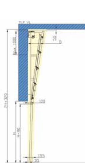
VL scorrimento verticale
